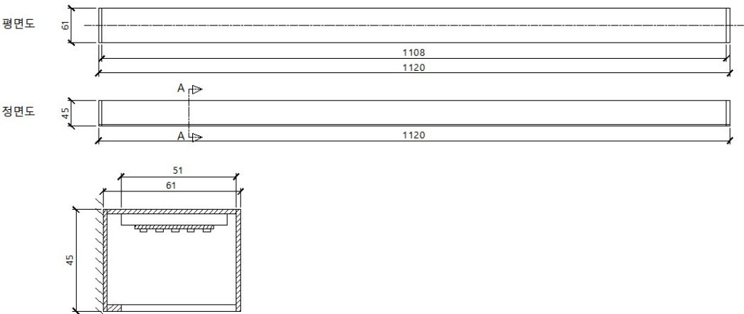
제품도면 (Unit: mm)
